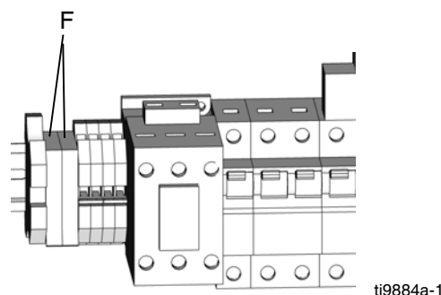
FIG. 4. Fusibles de ventilateur
