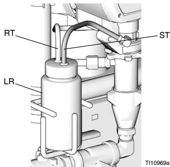
FIG. 10. Système de lubrification de la pompe
