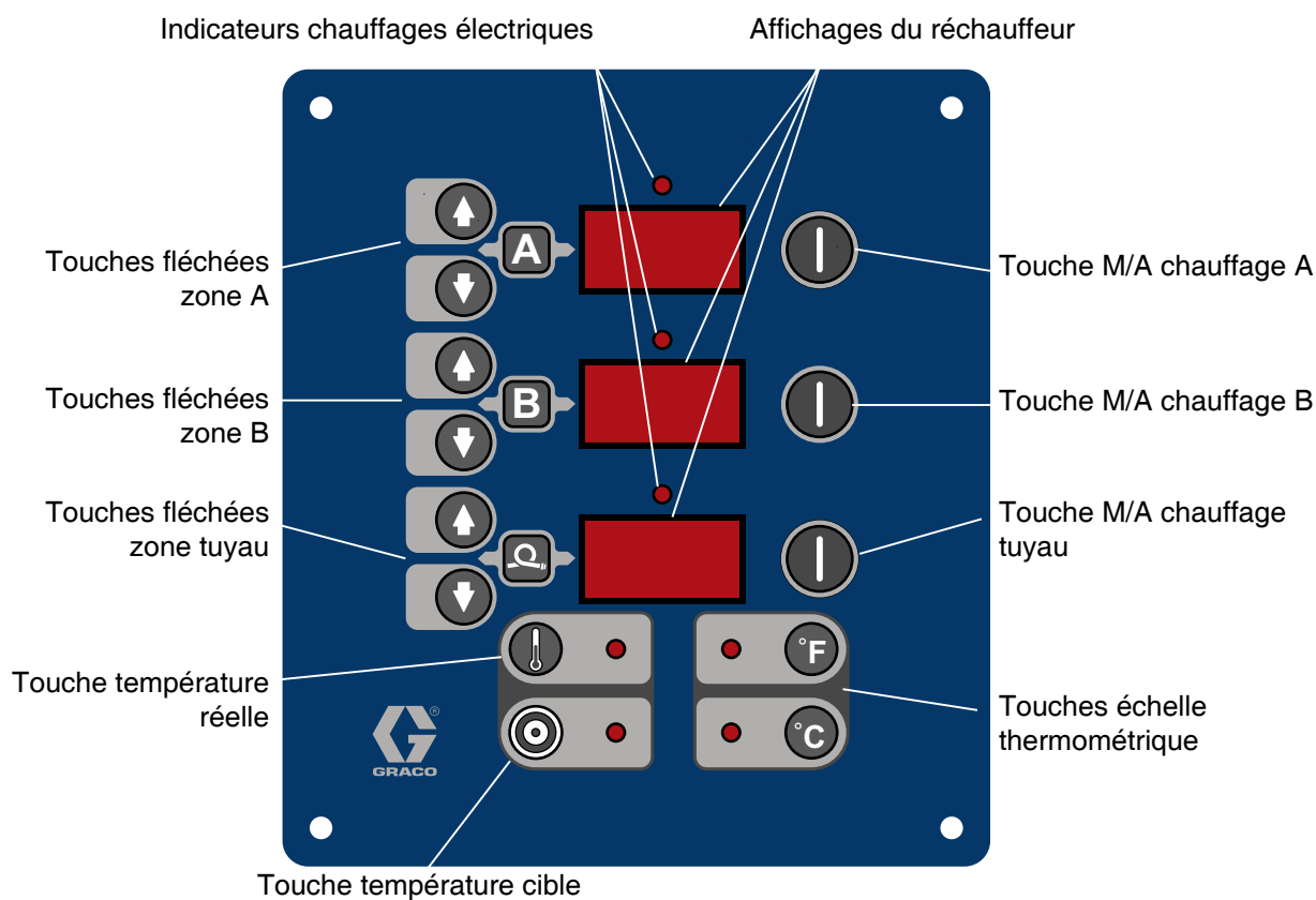
FIG. 4. Réglages et indicateurs de température
